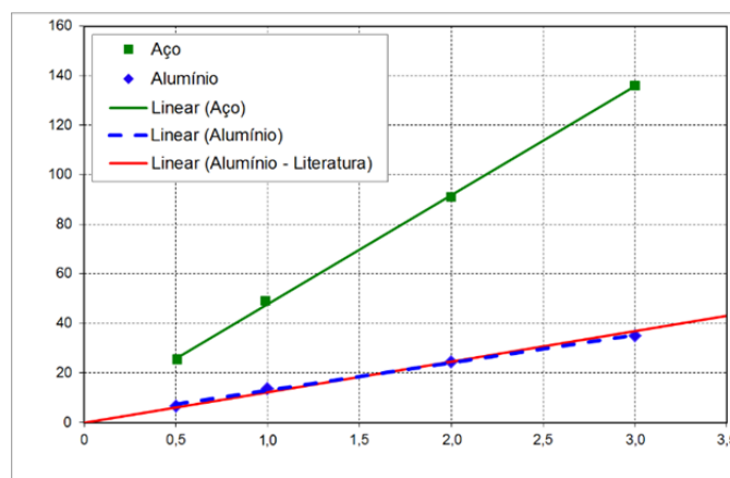
Fig. 2. Valores de tensão elétrica medidos nas amostras de aço e alumínio e comparação com os valores esperados para o alumínio segundo o valor teórico de condutividade elétrica.
