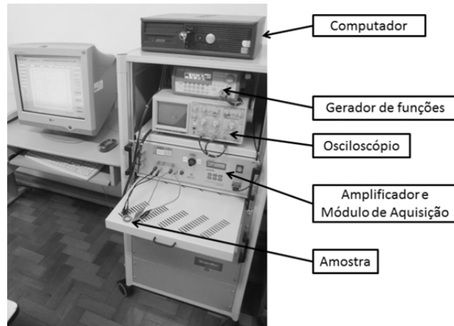
Fig. 4. Histeresígrafo TCH5000.
