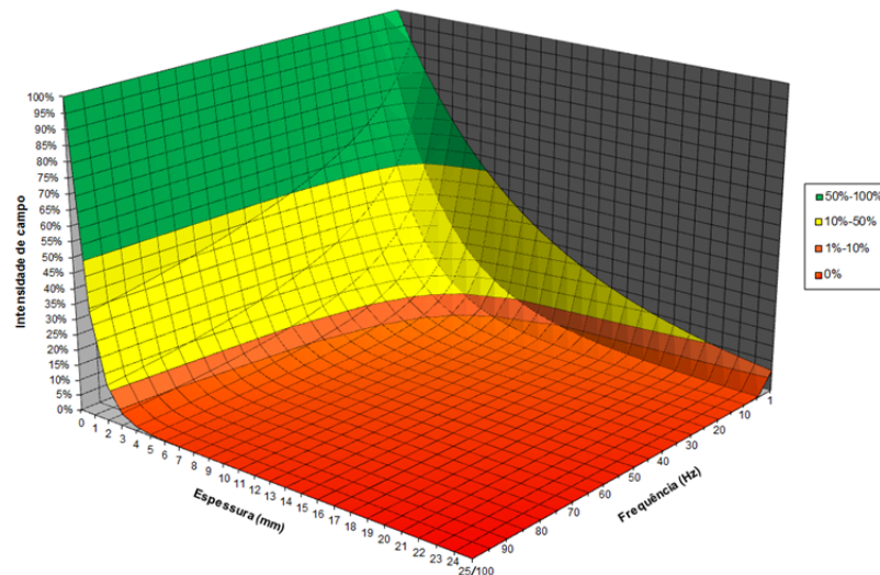
Fig. 7. Intensidade de campo que atravessa o aço em função da espessura e frequência.
